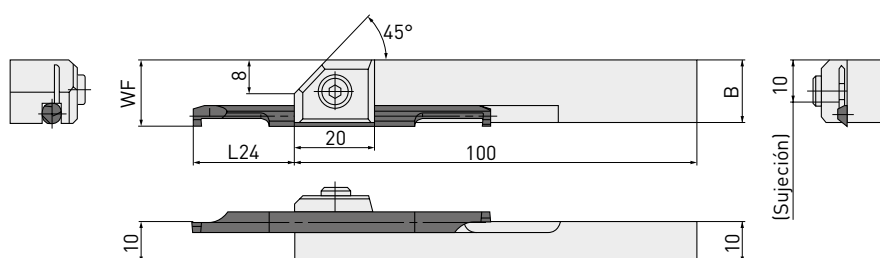
Tipo CG (la barra se acopla a portaherramientas)
